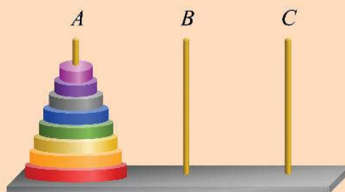
Hình 1. Mô hình Tháp Hà Nội với n = 8
